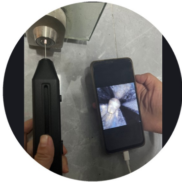
门锁内部查看
